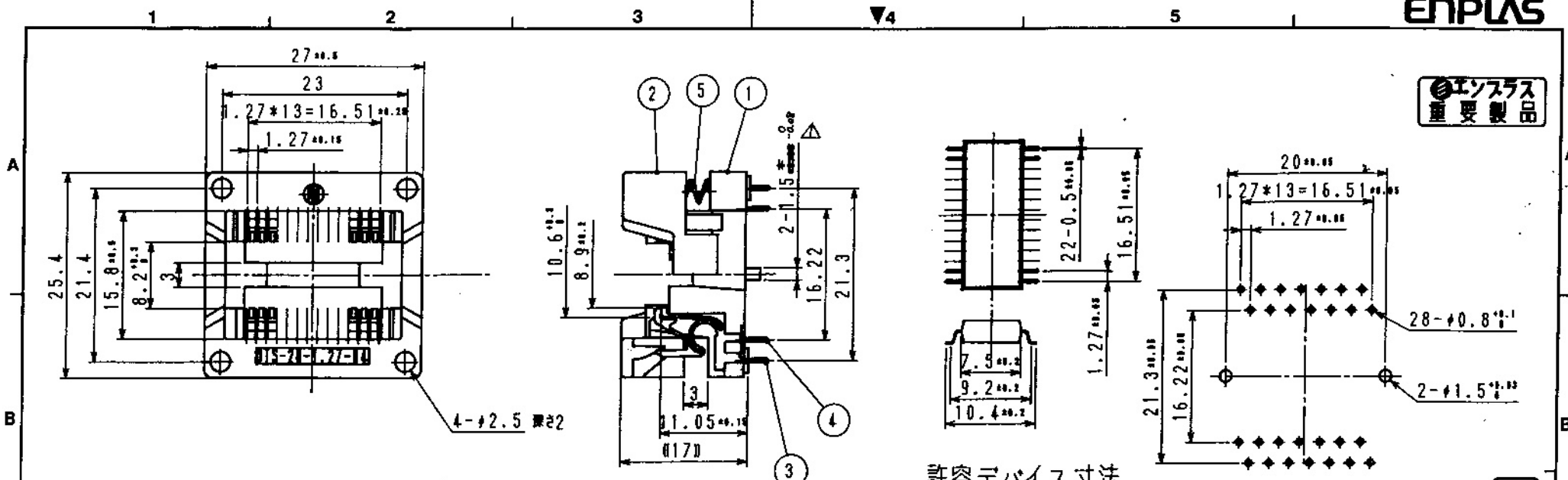
プリント基板裏面引付穴位置 (TOP VIEW) P.C.B. PATTERN
