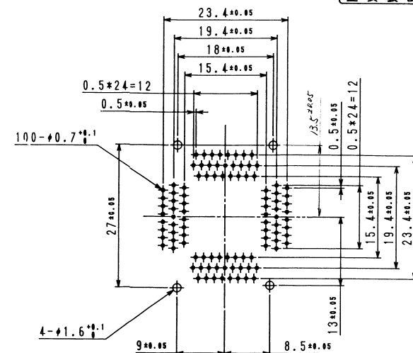
プリント基板取付け穴位置 (TOP VIEW) (2:1)
