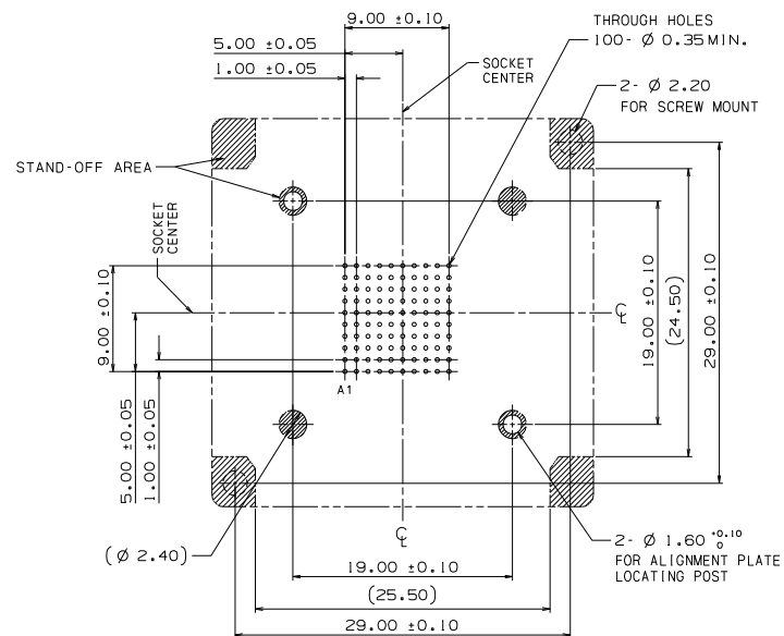
PCBホールパターン参考図(ソケット実装面側) PCB HOLE PATTERN(SOCKET SIDE/TOP VIEW)
